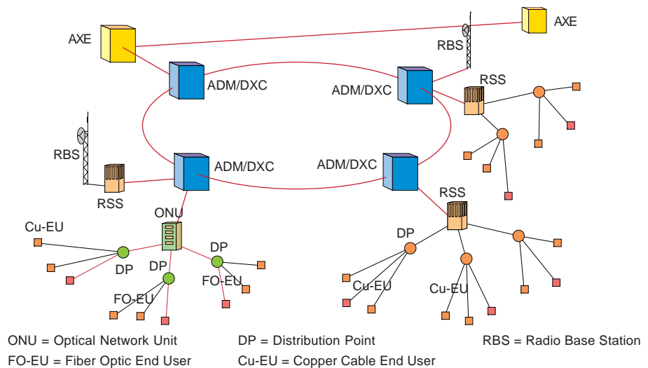
Fig 1-14. Optical fiber SDH ring with AXE, ADM/DXC, RSS och RBS
