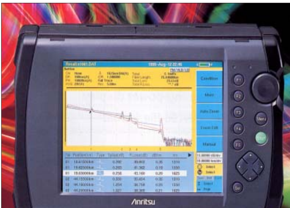
Fig. 10-1 Portable OTDR. Photo courtesy of Anritsu Inc.
